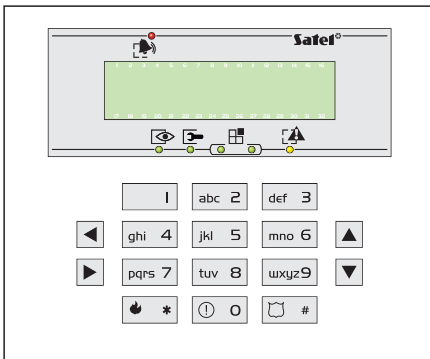
Rys. 2. Widok manipulatora INT-KLCDS-GR.
